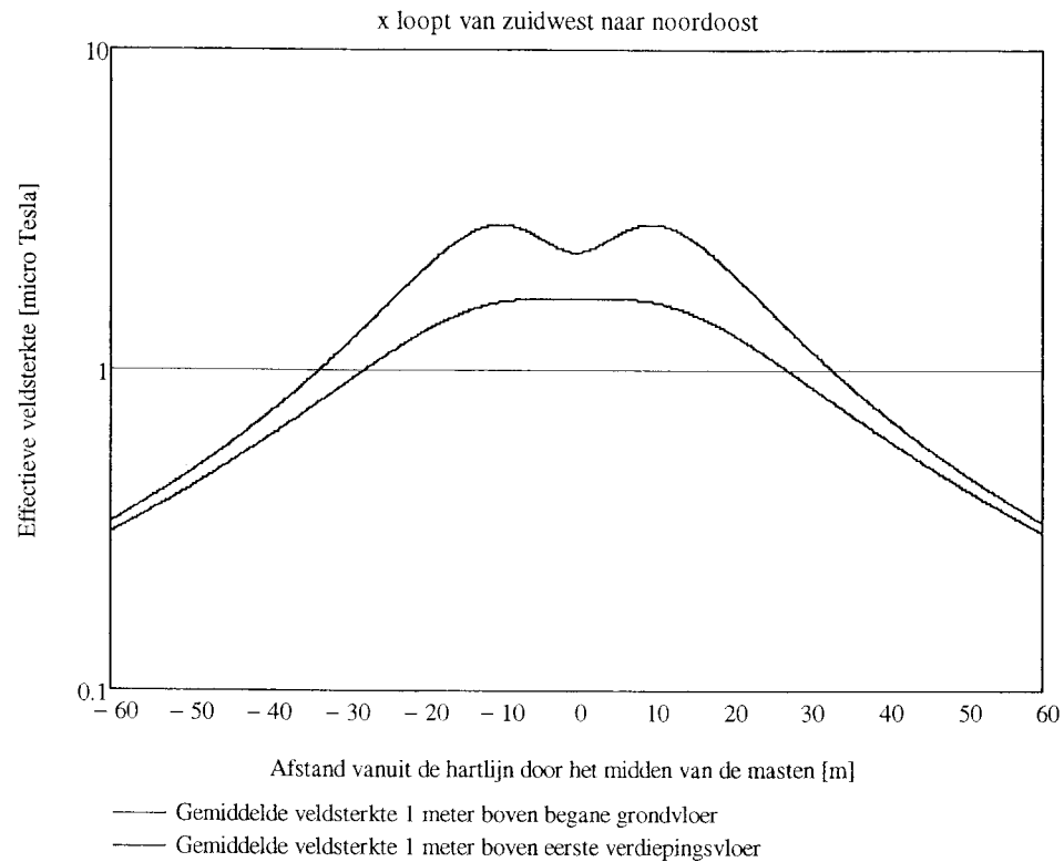
Figuur 6 Veldsterkteberekening volgens de methode voor specifieke zone maar op 1 meter boven de vloer van de begane grond en eerste verdieping.
